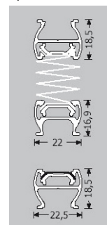
Cotes des profils
