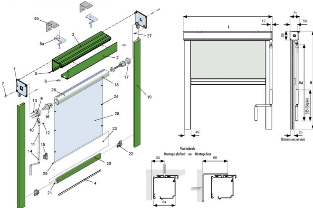
Schéma du store coffre 63 avec manoeuvre à treuil/manivelle et coulisses latérales
