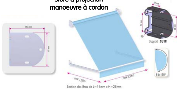
Section des Bras de L=11mm x H=25mm
