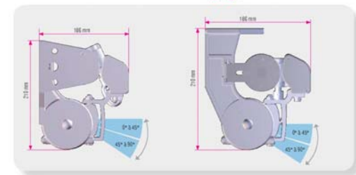
Tension des bras par double câble gainés pour tous les stores
